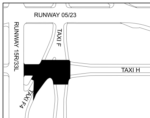
Figure 3 : Zone de travaux de la voie de circulation H et de la voie de circulation F
