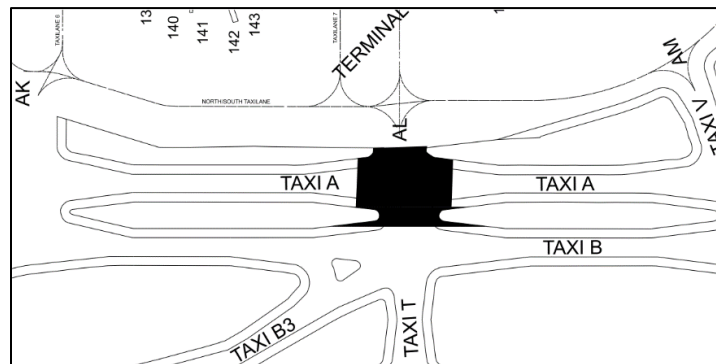
Figure 18 : Zone de travaux sur la voie de circulation A, phases 3 et 3A
