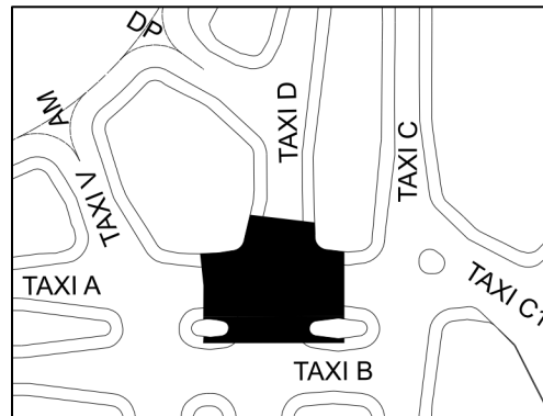
Figure 16 : Zones de travaux sur la voie de circulation A, phases 1 et 1A
