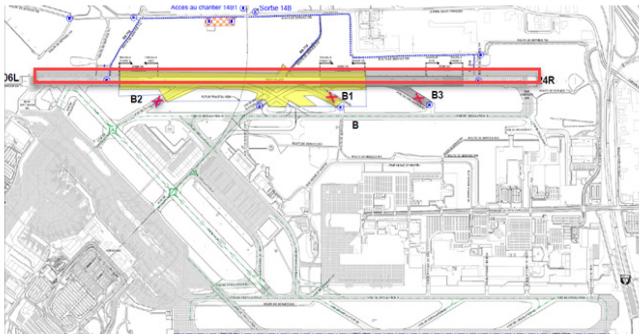
Figure 1 : Piste 06L/24R – Travaux de construction
